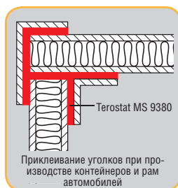
Terostat MS 9380
